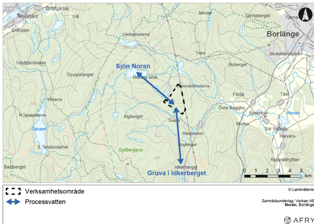
Figur 9-1 Schematisk bild över de två vattentäkter som utreds för försörjning av processvatten till verksamheten.
